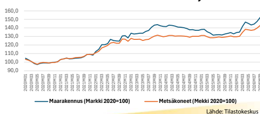
Konekustannusindeksien kehitys
